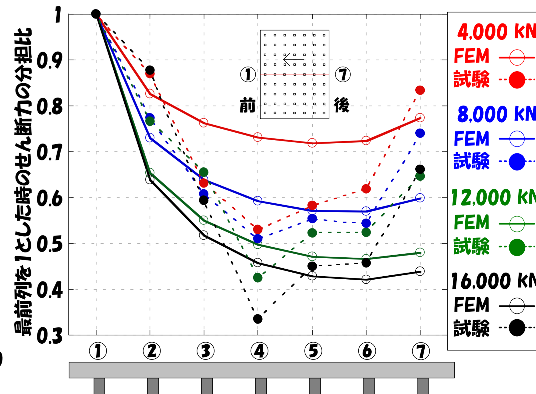
各杭のせん断力の分担の違い
