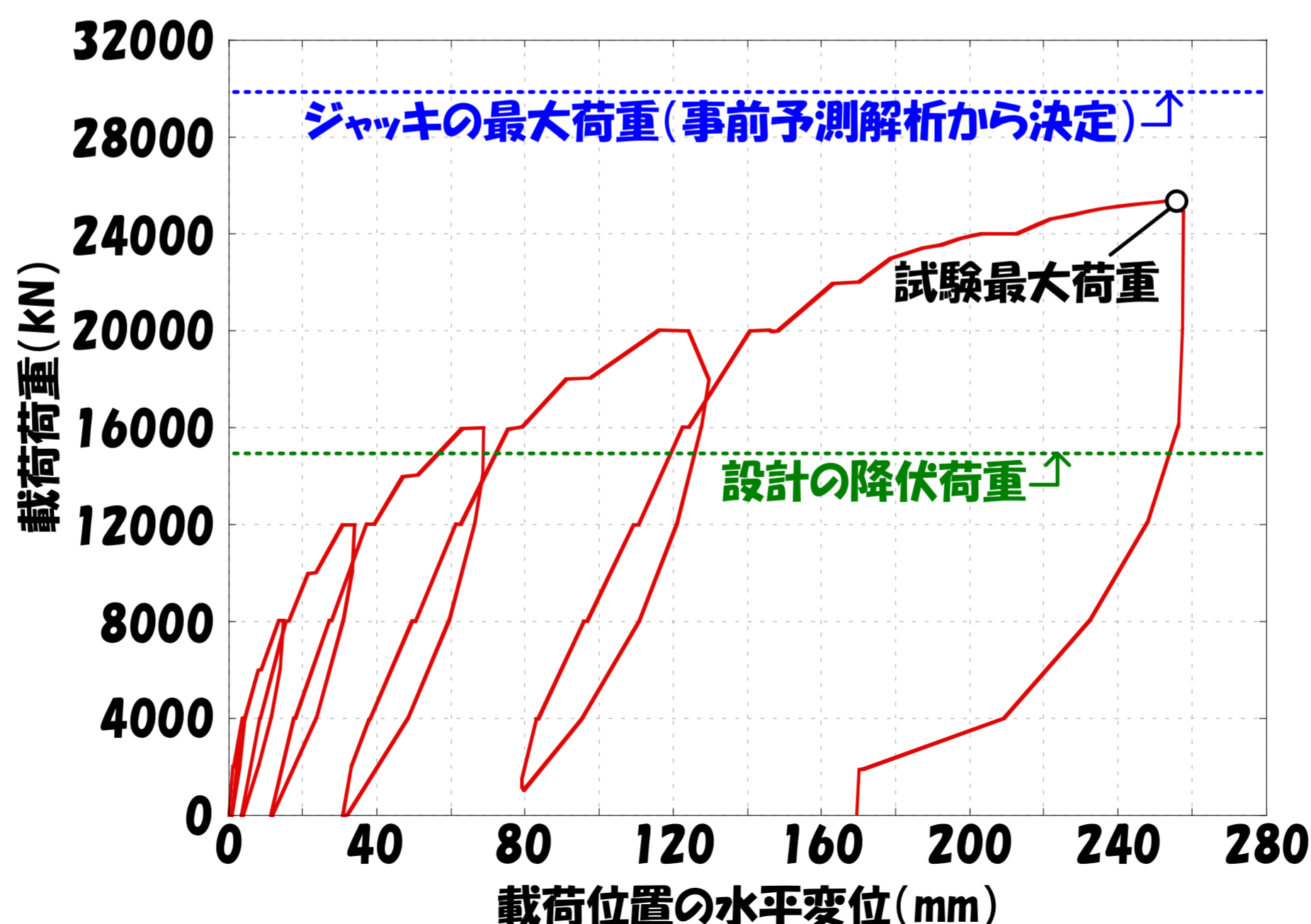
荷重 - 変位関係と耐力照査
